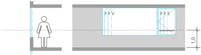
1-Meter-Regel: Absturzhemmung durch Verbund-Sicherheitsglas (V) und Personenschutz durch Sicherheitsglas (S)
