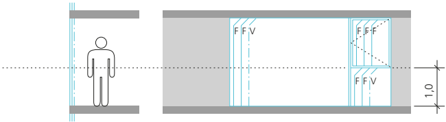
Absturzhemmung durch Verbund-Sicherheitsglas (V)
